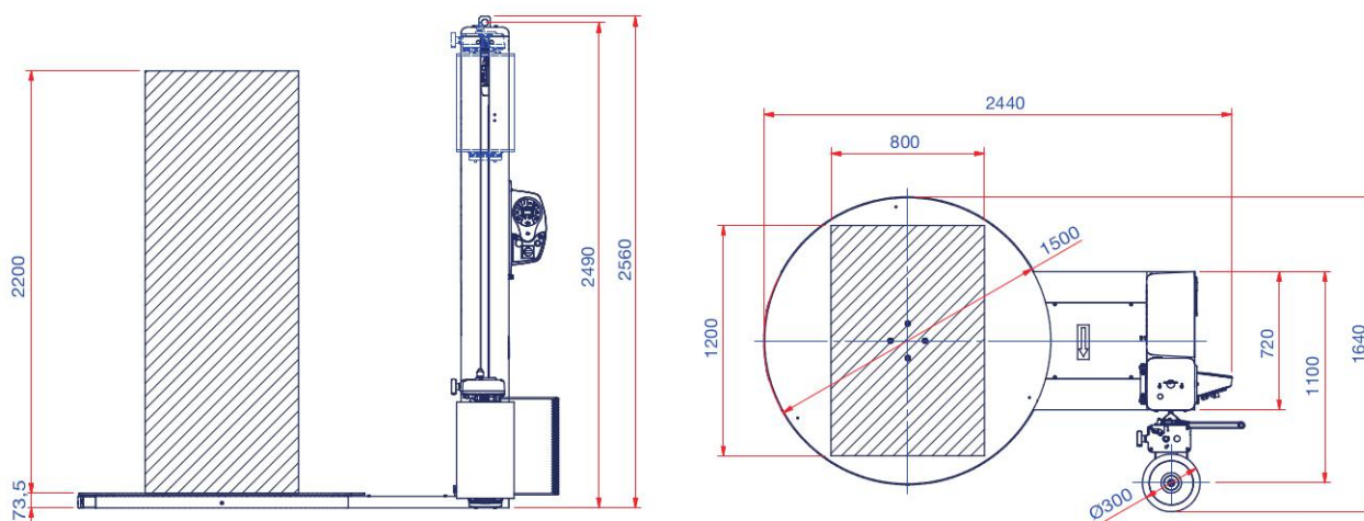
ΤΕΧΝΙΚΟ ΣΧΕΔΙΟ ECOPLAT FRD [mm] СХЕМА НА ECOPLAT FRD [mm]
